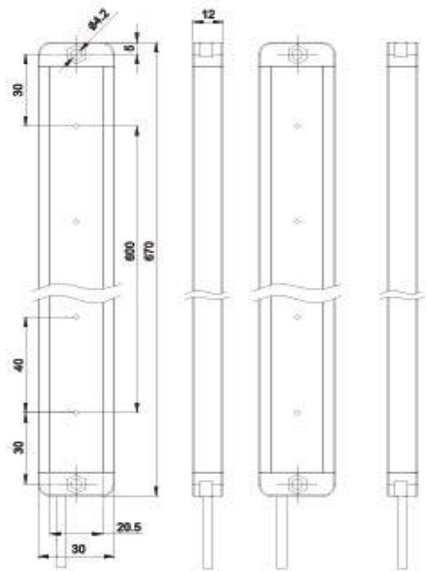
XH16-2M□-U5-40
