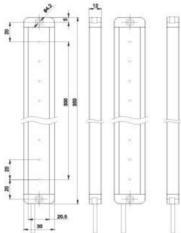
XH16-2M□-U5
