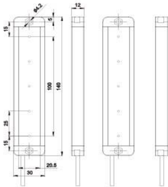
XH5-2M□-U5
